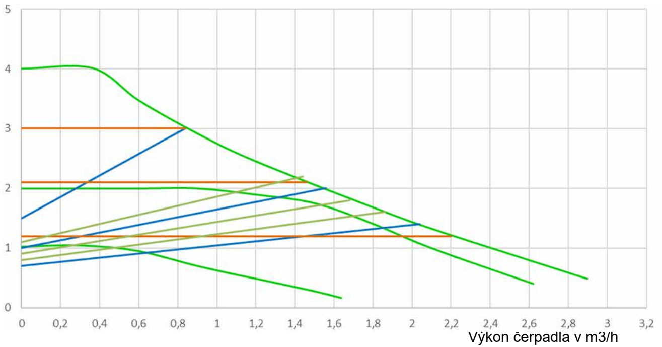
6.4 Výkonové charakteristiky CPH 2.0 40/XXX
