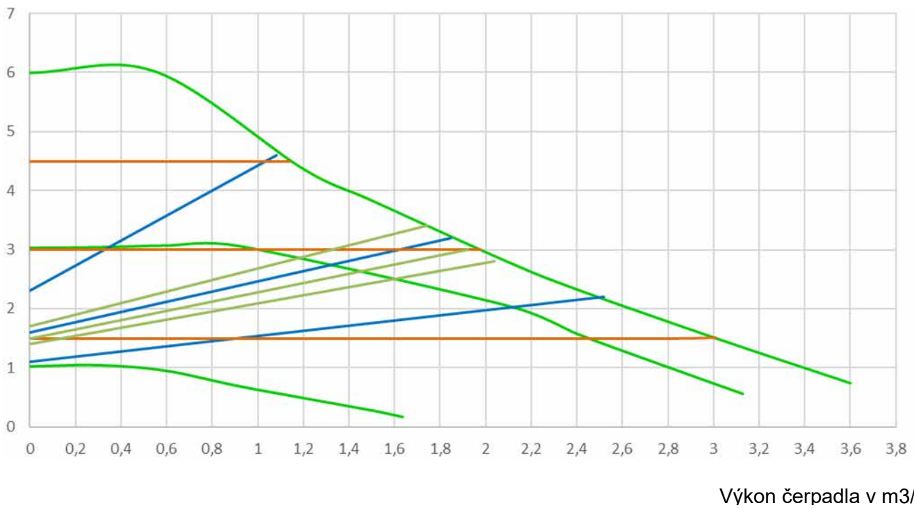
Dopravní výška v m CPH 2.0 60/XXX
