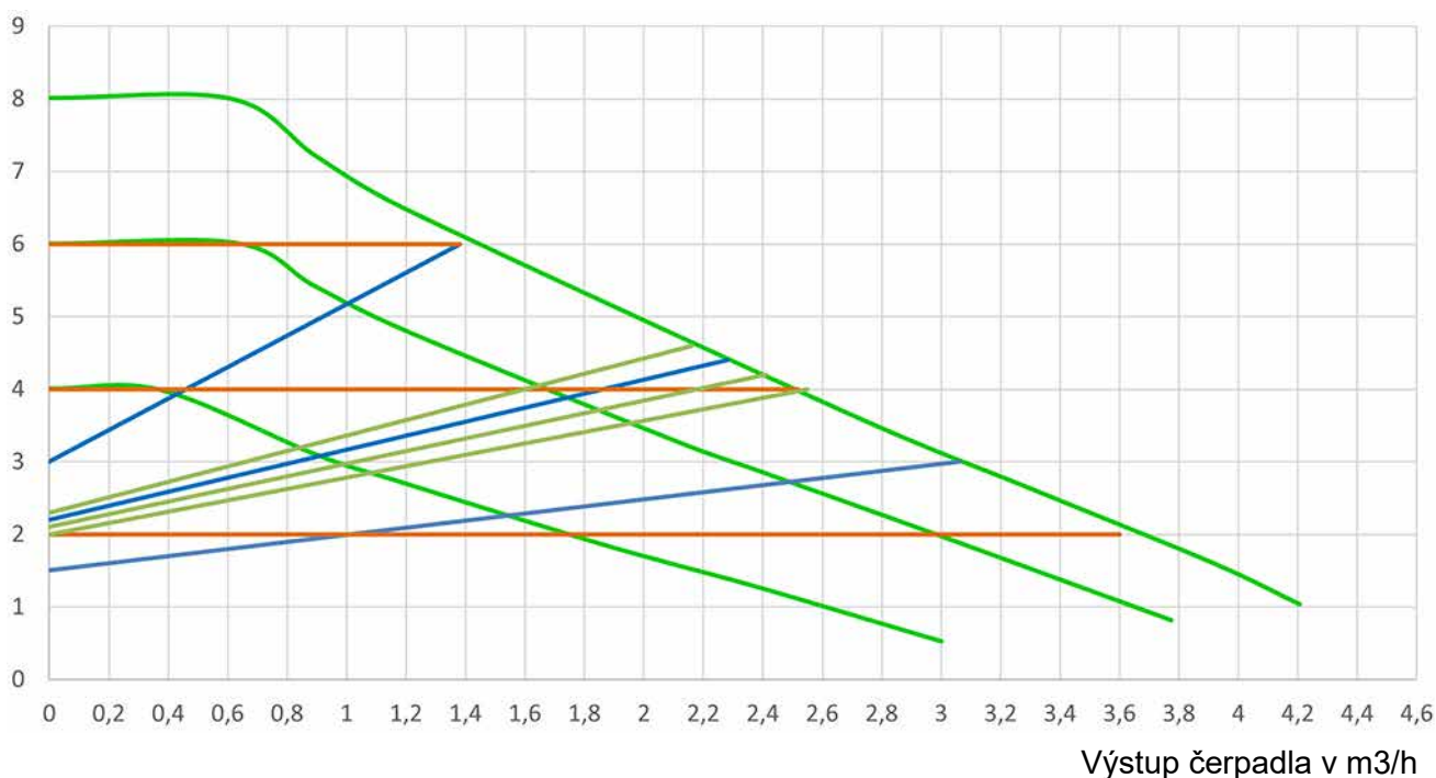
Dopravná výška v m CPH 2.0 80/XXX
